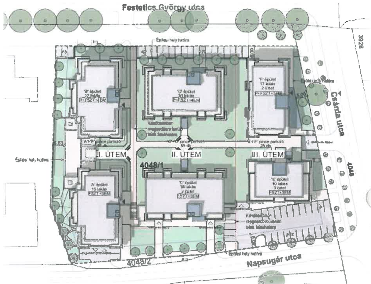
a tervezett beruházás helyszínrajza
