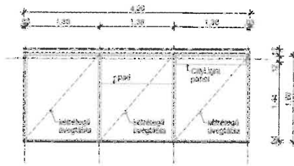
FELÜLNÉZET
