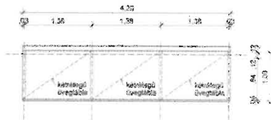
FELÜLNÉZET
