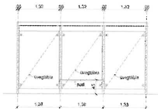
ELÜLNÉZET
